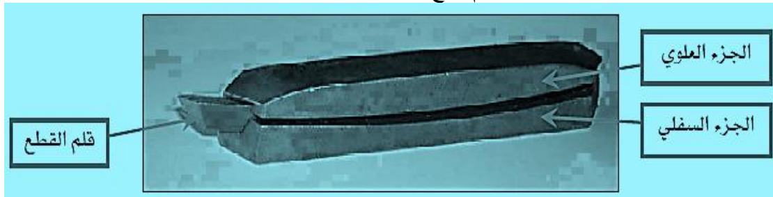
ج. لقم من فولاذ السرعة العالية مثبت بمربط
