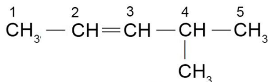
4 - مثيل - 2 - بنتين
