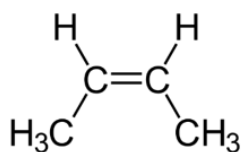
سس -2- بيوتين
