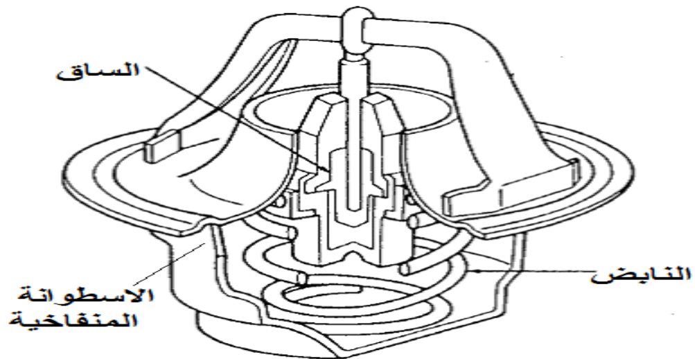
أجزاء المنظم الحراري
