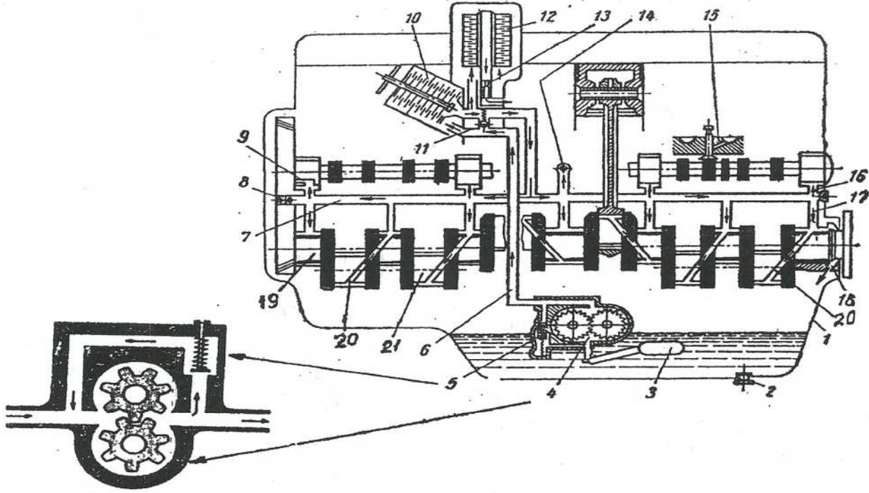
جهاز تزييت المحركات المركب
