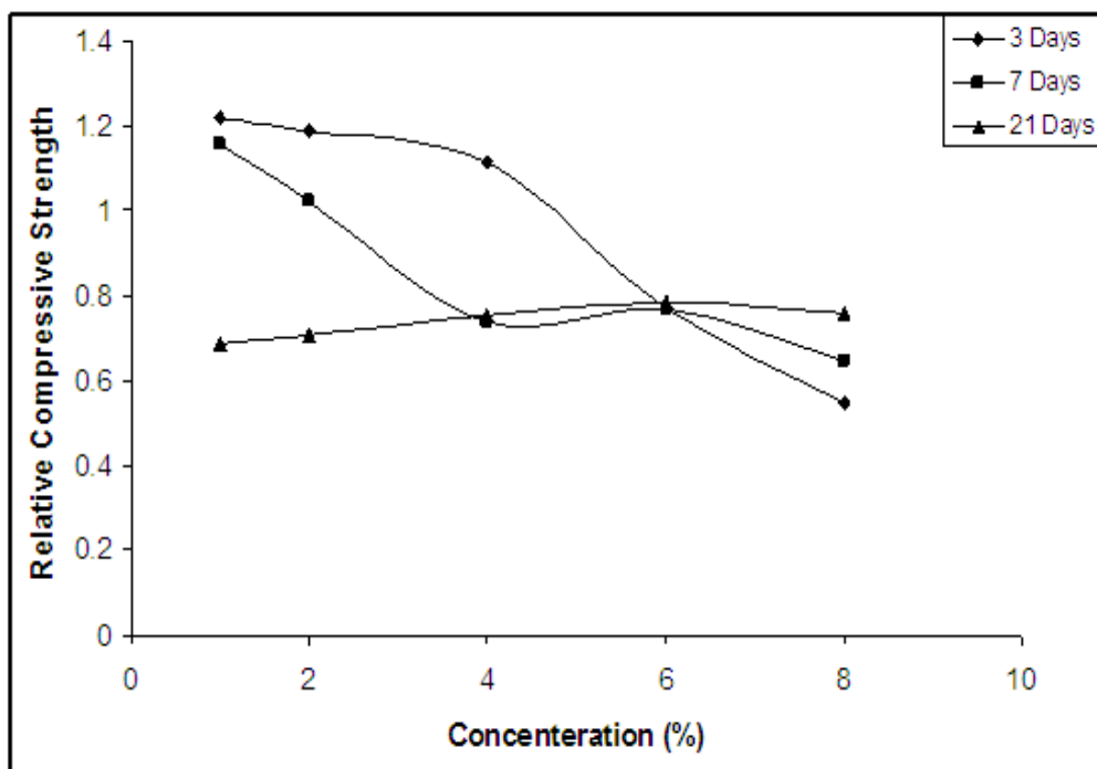
الشكل (4): يوضح التغير في مقاومة الانضغاط النسبية مع نسبة المضاف.
