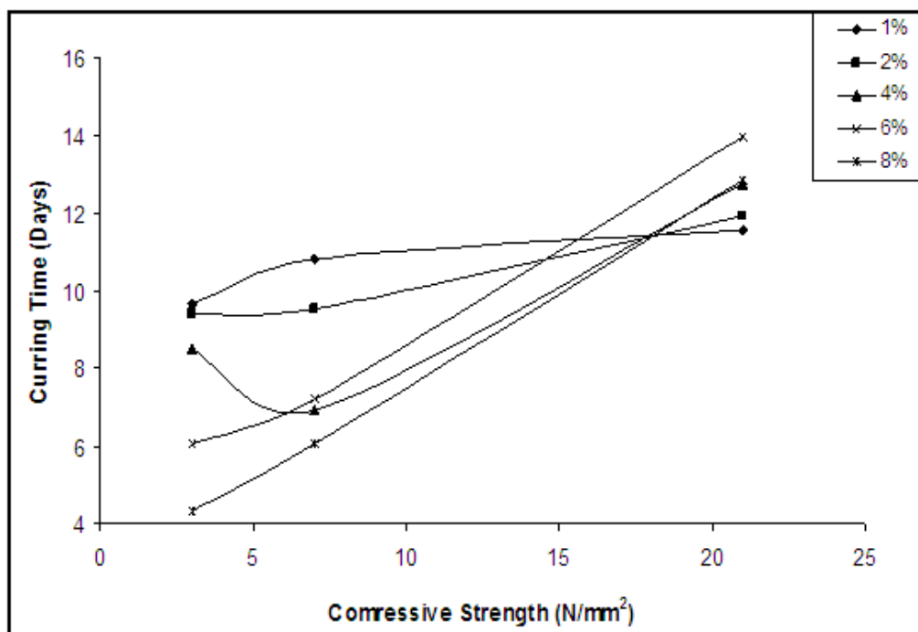
الشكل (5): يوضح التغير في مقاومة الانضغاط مع زمن المعالجة بالرطوبة.
