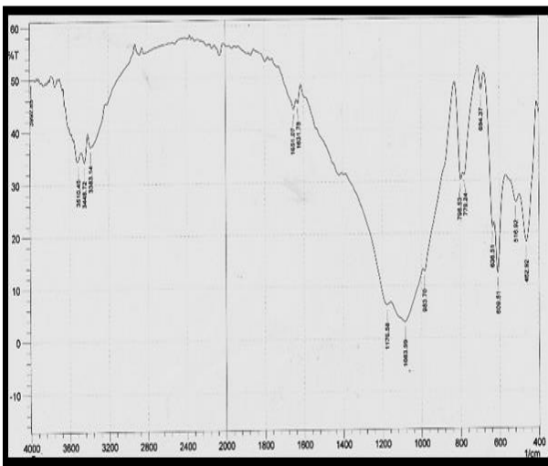
Fig.(17):FTIR spectra for bentonite
