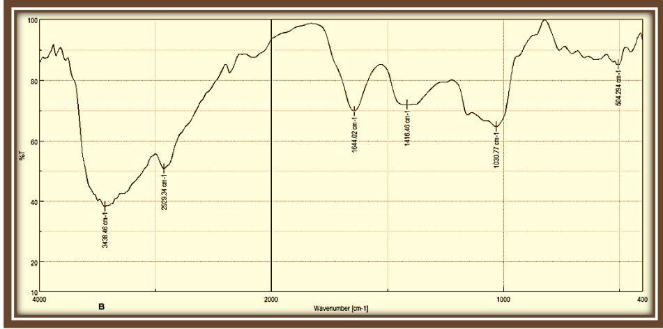
شكل (6): مرسم طيف الأشعة تحت الحمراء للبيتاكلوكان المستخلص من نخالة الشعير الاسمر
