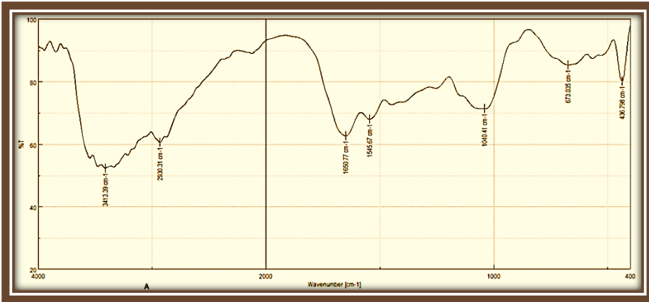
شكل (5): مرتسم طيف الاشعة تحت الحمراء للبيتاكلوكان المستخلص من خميرة الخبز
