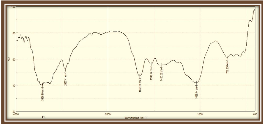
شكل (4): مرتسم طيف الاشعة تحت الحمراء للبيتاكلوكان القياسي
