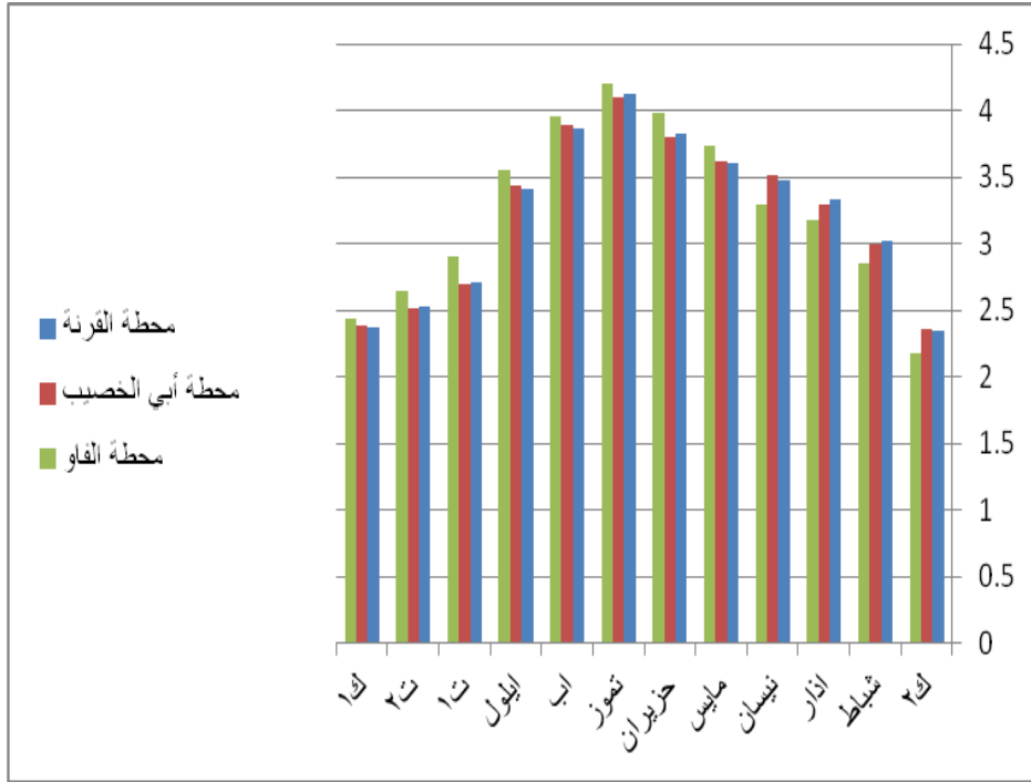
شكل ( ٦ ) المعدلات الشهرية والسنوية لسرعة الرياح ( م / ث ) في محطات منطقة الدراسة للمدة ( ٢٠١٤ - ٢٠١٩ ) .
